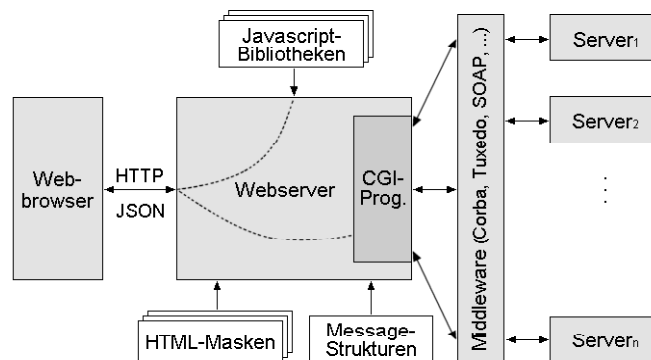
Abbildung 5: Architektur des Zielsystems
